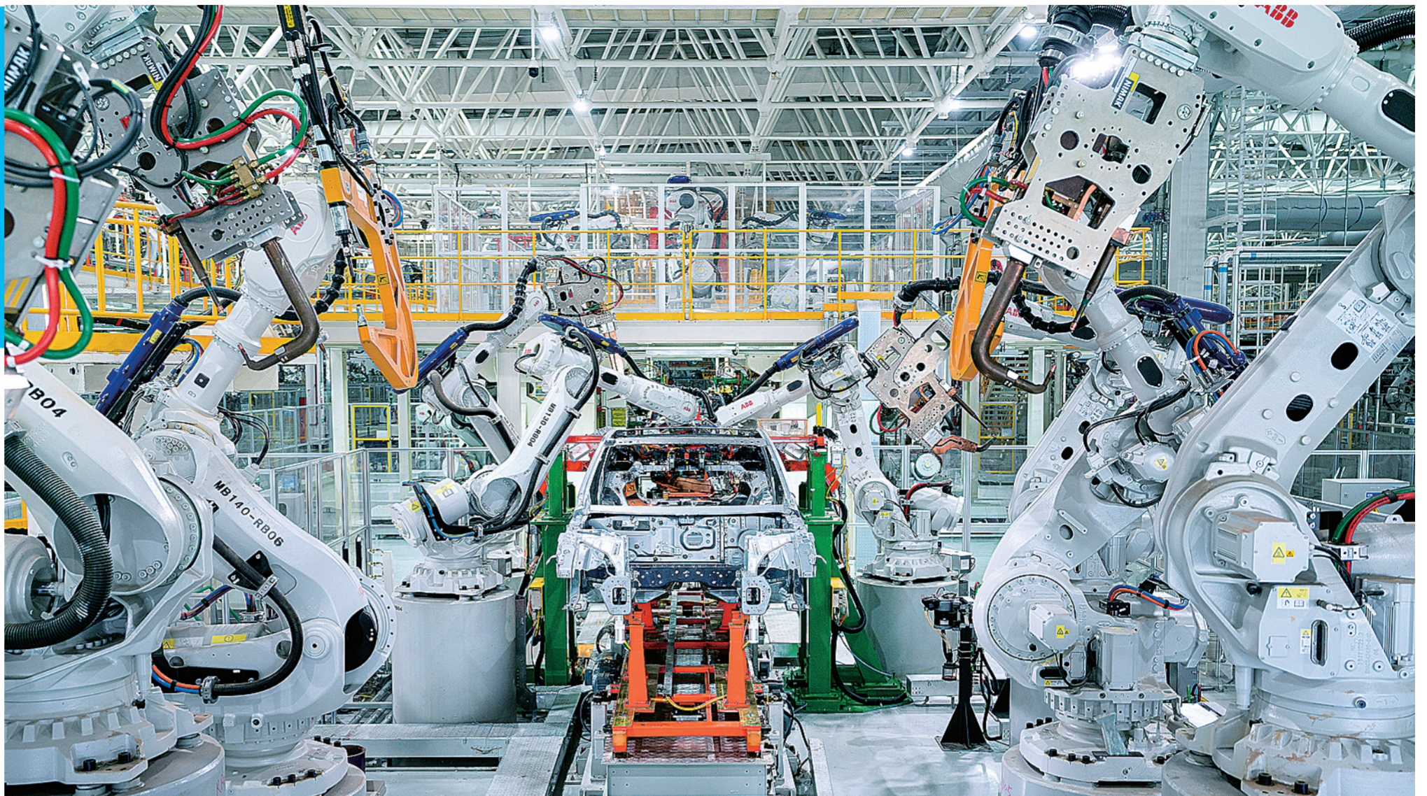
肇庆小鹏汽车智能网联科技产业园，厂区共设有冲压、焊装、涂装、总装、Pack五大车间，拥有4种不同车型总装柔性生产线及1条柔性电池合装线，共计设置264台智能工业机器人。
